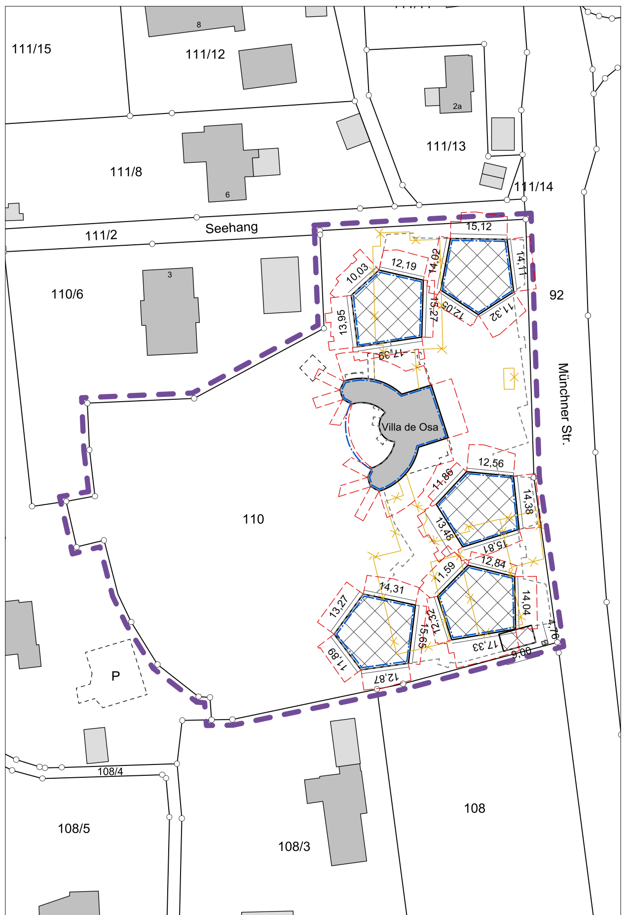
Lageplan M 1:1000
